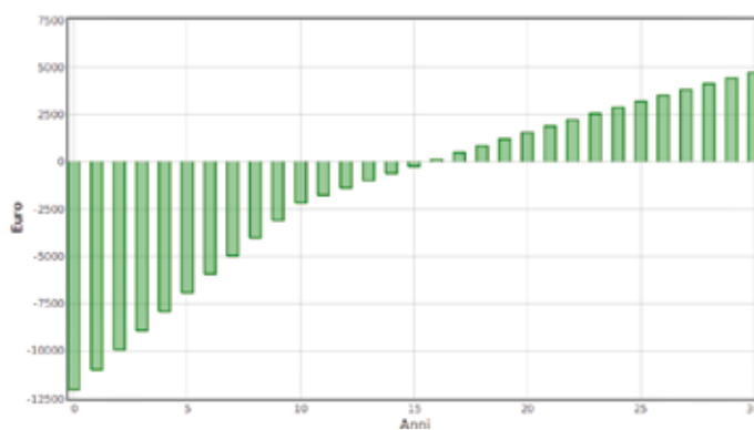
Stima del risparmio economico generato dalla sostituzione di 16 mq di serramenti anni '70 con serramenti da 1,3 W/m 2 K. e utilizzo Termosoglia e Coprisoglia
